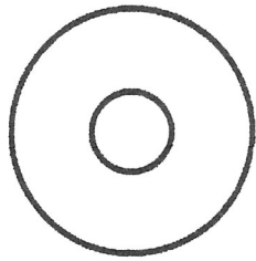
Circle Map
